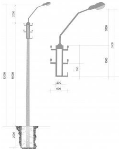
Опора из ж/Б
